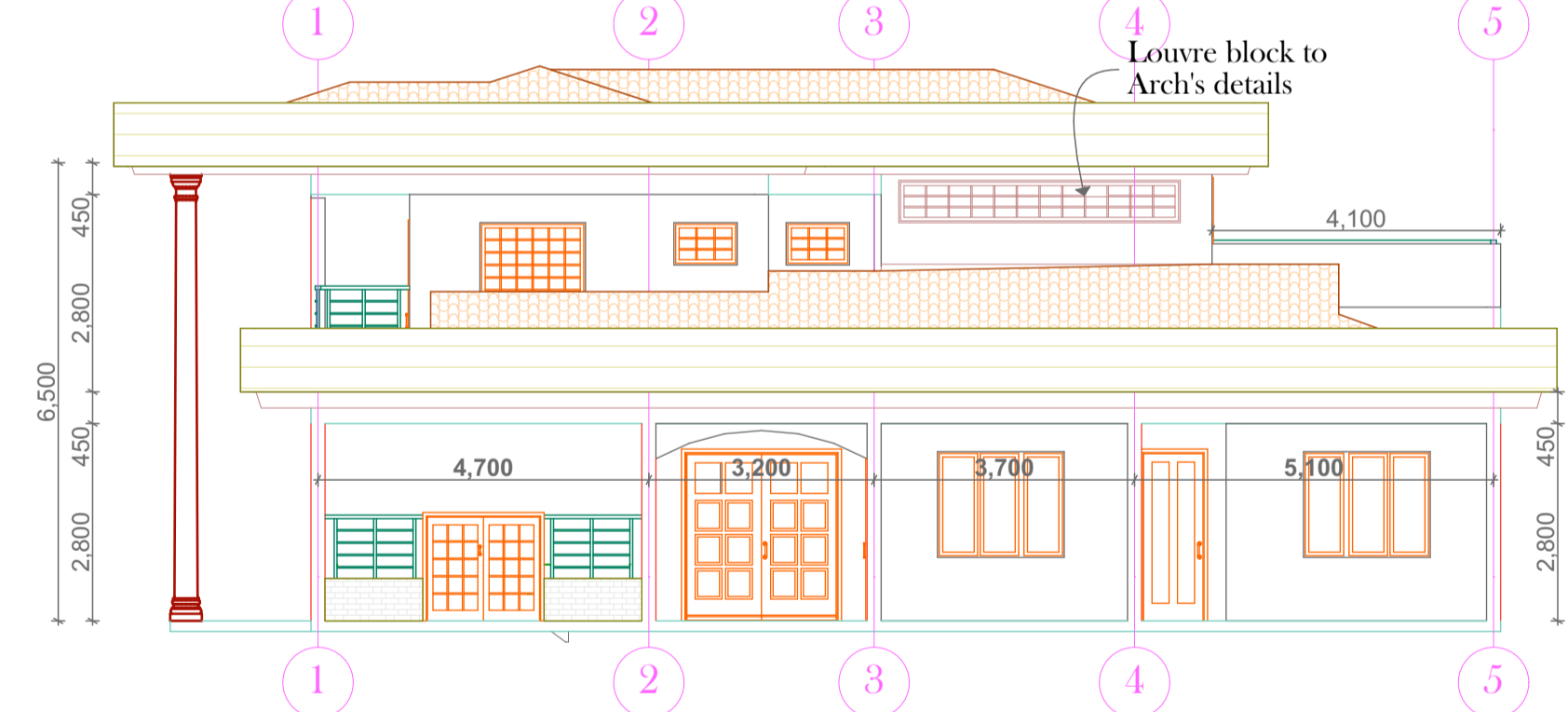
ELEVATION 02
