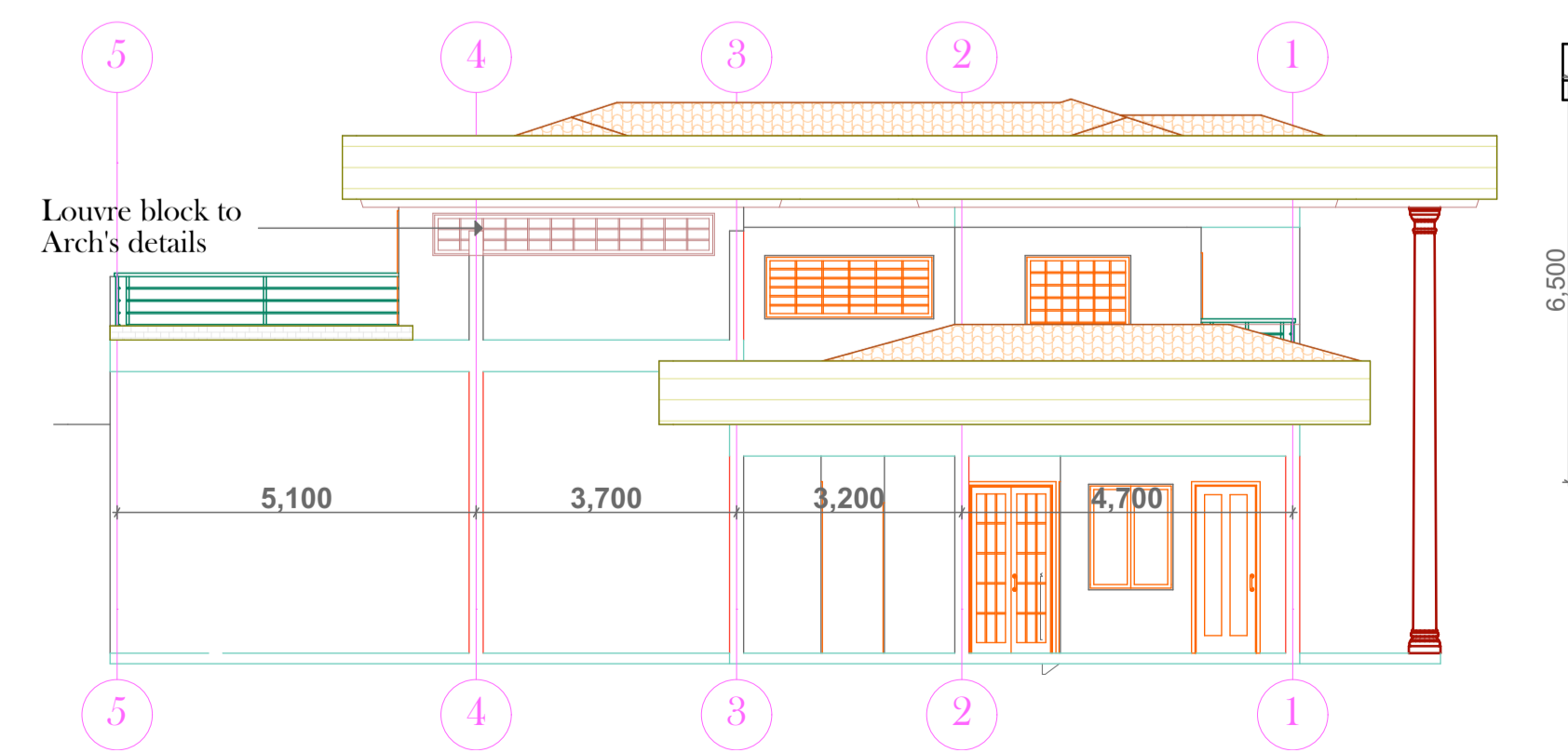
ELEVATION 04
