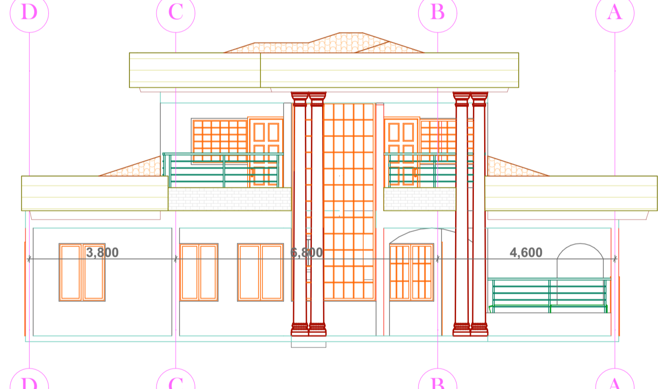
ELEVATION 01
