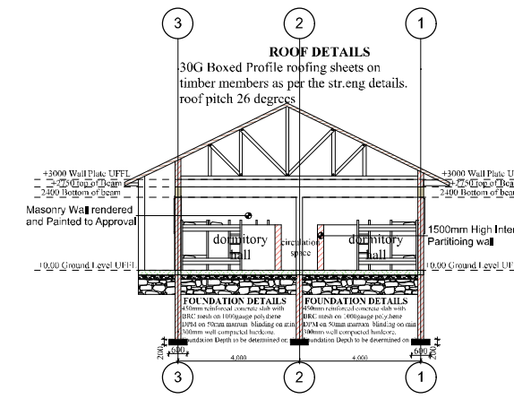
SECTION 01
